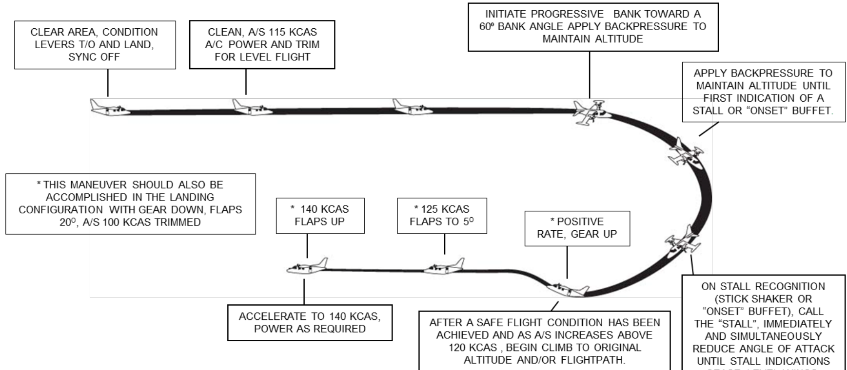
Figure C-11 MU-2B B, D (-10), F (-20), G (-30)
