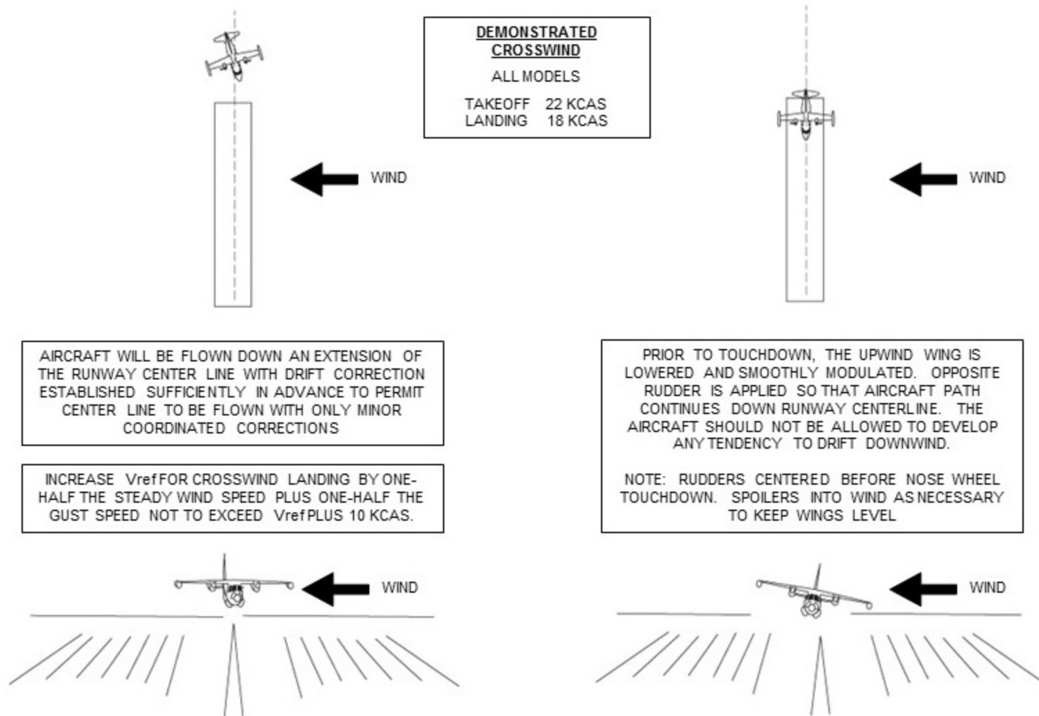
Figure A-20 MU-2B MARQUISE (-60), SOLITAIRE (-40), N (-36A), P (-26A) CROSSWIND LANDING
